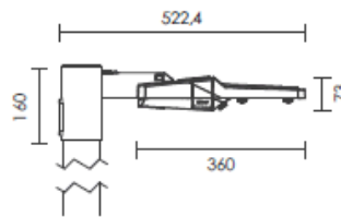
Lumina Mini 76mm SPIGOT Side View
